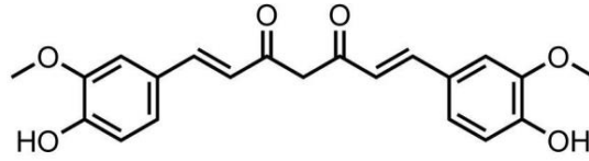
Şekil1. Kurkumin Kimyasal Yapısı (diferuloilmetan)
